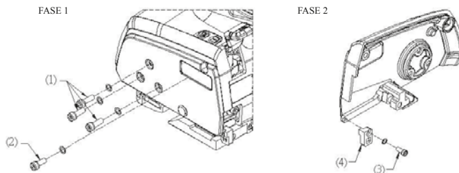
FIG. 8. Illustrazione della sostituzione della guida posteriore della reggetta
