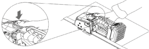
FIG. 13. Funzionamento tensione
